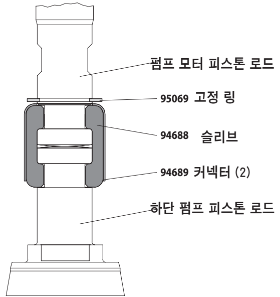
펌프 연결 세부도
